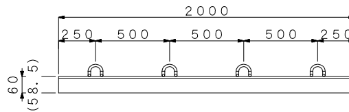
平面図 アンカーピッチ
