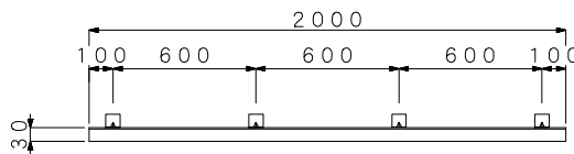
平面図 アンカーピッチ
