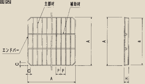
納まり図
