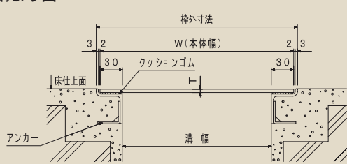
納まり図
