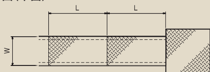
納まり図(平面)
