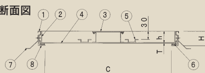
断面図
