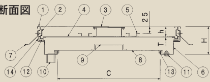
断面図
