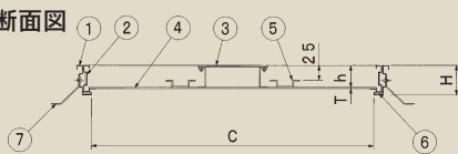
断面図
