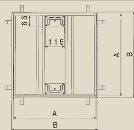
平面図
