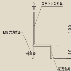
SISLU詳細図
