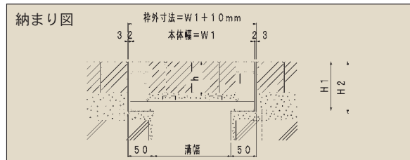
※受枠アンカーは、図表仕様になります。
