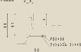
排水部目地詳細図
