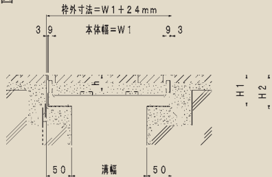
●SH-2(インサート取手) ※材質SUS304
