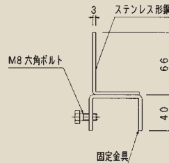
SOSLU詳細図
