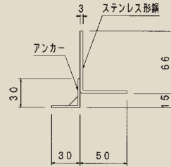
SOSL詳細図
