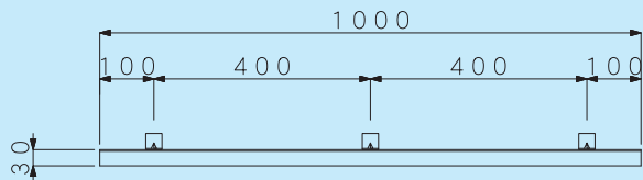
平面図 アンカーピッチ
