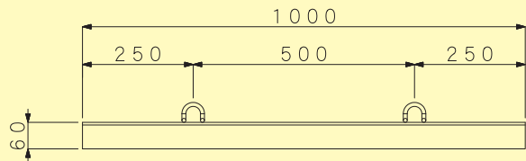
平面図 アンカーピッチ
