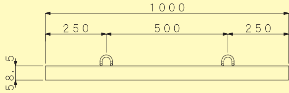
平面図 アンカーピッチ
