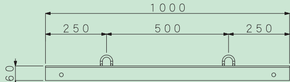
平面図 アンカーピッチ
