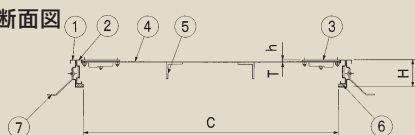
断面図
