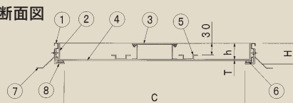
断面図
