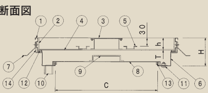
断面図
